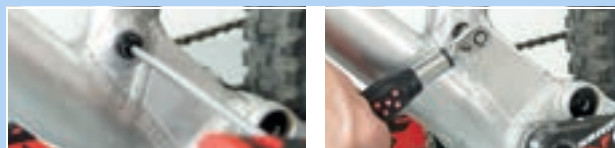
Abbildung 178: Postpin Achse befestigen
