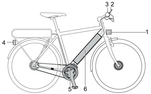
Abbildung 29: Schema Elektrisches Antriebssystem
