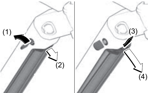
Abbildung 118: Akku herausnehmen
