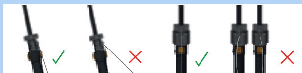
Abbildung 175: Korrekter und falscher Bowdenzug
