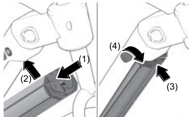
Abbildung 119: Akku einsetzen
