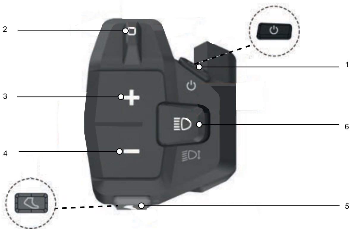
Abbildung 41: Übersicht Bedieneinheit BOSCH
