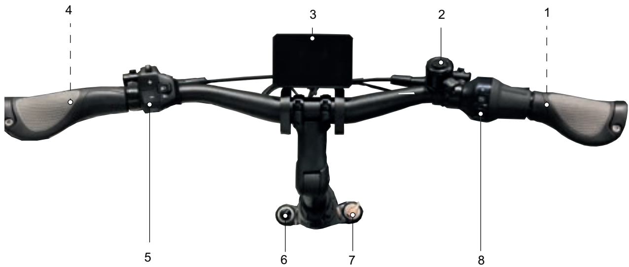
Abbildung 33: Detailansicht Lenker mit SHIMANO SC-E800 Bordcomputer, Beispiel
