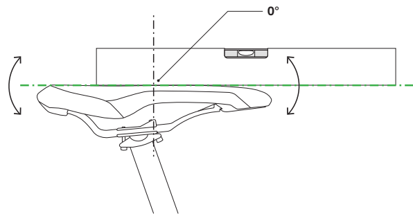
Abbildung 82: Waagerechte Sattelneigung mit 0° Neigung in der Sattelmitte
