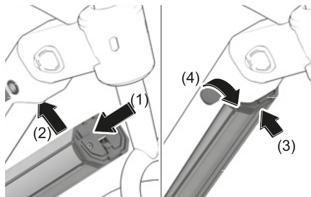
Afbeelding 49: Geïntegreerde accu aanbrengen
