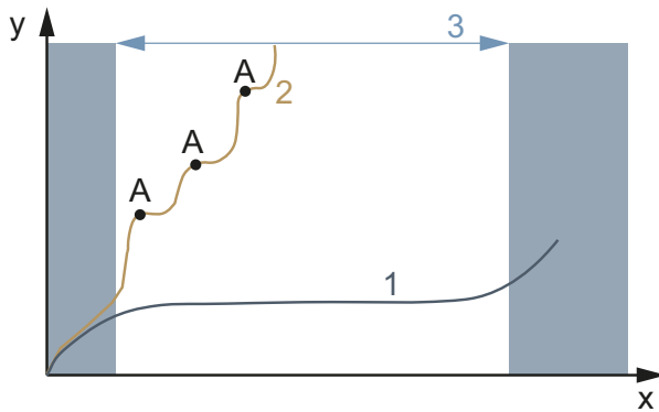
Afbeelding 146: Grafiek slijtage, bedrijfsduur (x) tegen materiaalaafname (y)
