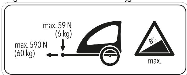
Afbeelding 129: Waarschuingssticker aanhanger
