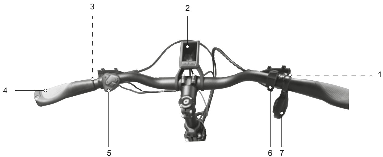
Afbeelding 39: Detailaanzicht stuur met BOSCH Kiox boordcomputer, voorbeeld
