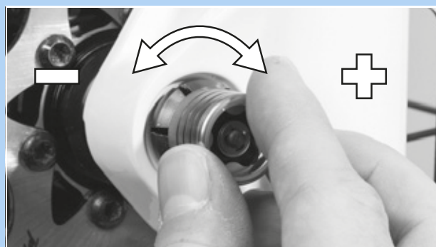
Afbeelding 79: Spanning afstellen
