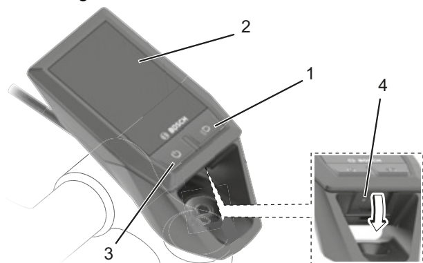
Afbeelding 40: Opbouw BOSCH Kiox boordcomputer
