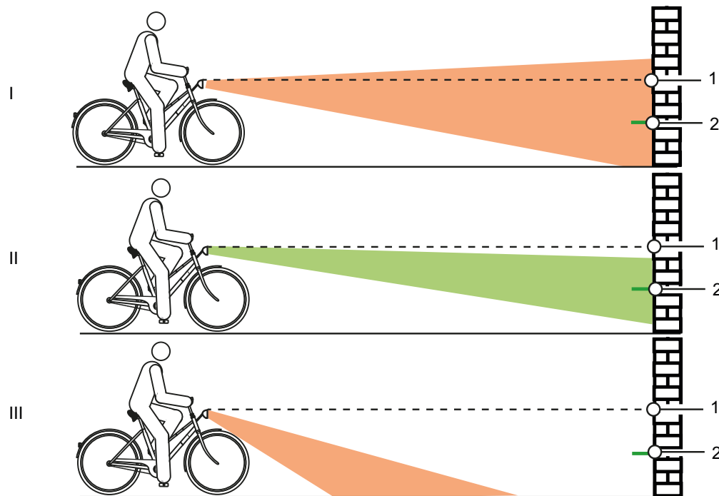
Afbeelding 153: Te hoog (1), correct (2) en te laag (3) afgestelde verlichting
