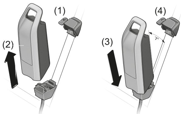
Afbeelding 136: Frame-accu verwijderen en aanbrengen
