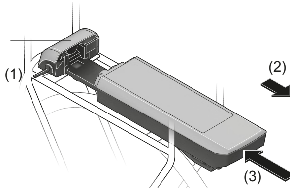
Afbeelding 47: Bagagedrageraccu verwijderen (2) en aanbrengen (3)
