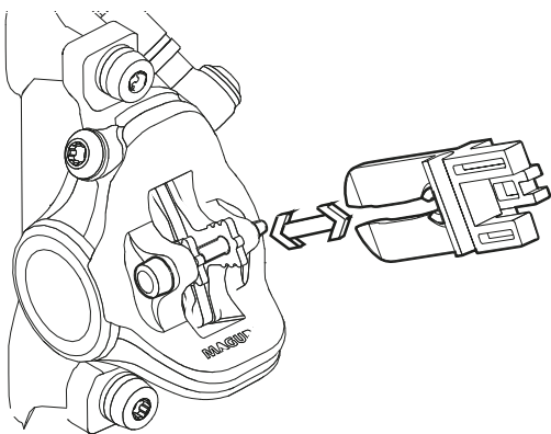
Afbeelding 51: Transportbeveiliging bevestigen
